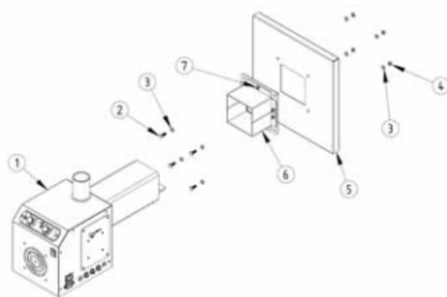
Εικ.10β. 'B-ECO 3 Εγκατάσταση
