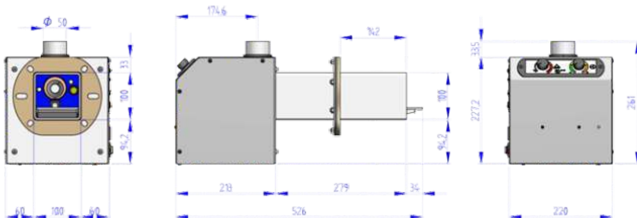
Εικόνα. 5a². 'B-ECO 2 (² Με τετράγωνο θάλαμο καύσης)
